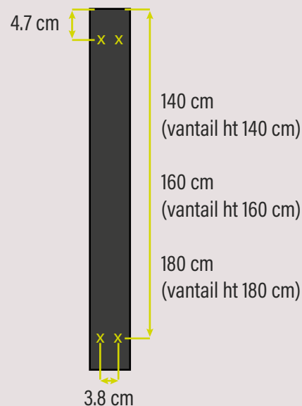
Schéma de perçage Poteaux de portail aluminium
