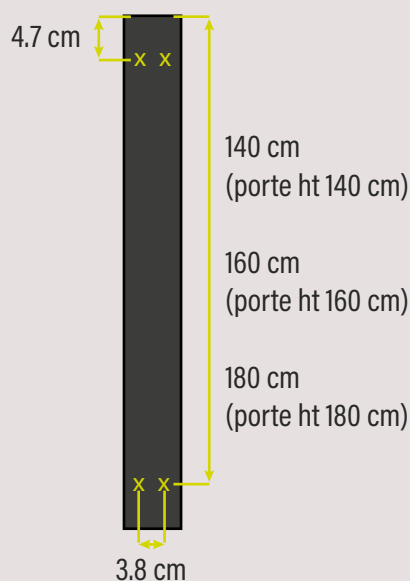
Schéma de perçage Poteaux de portillon aluminium
